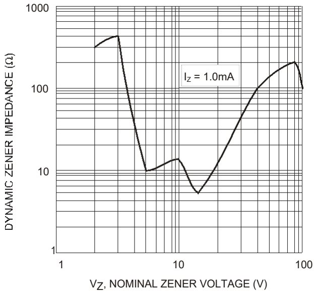
Fig. 1 Zener Voltage vs. Zener Impedence
